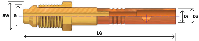
G: Schroefdraad, SW: Sleutelbreedte, Da: Buitendiameter, Di: Binnendiameter, LG: Totale lengte
