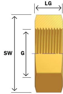
G: Schroefdraad, SW: Sleutelbreedte, LG: Hoogte
