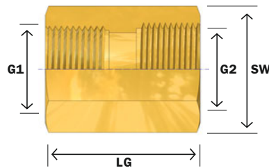
G: Schroefdraad, SW: Sleutelbreedte, LG: Totale lengte
