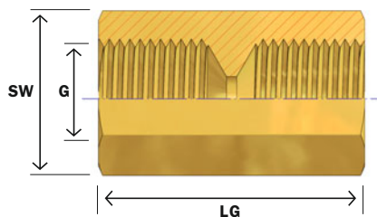
G: Schroefdraad, SW: Sleutelbreedte, LG: Wartel lengte
