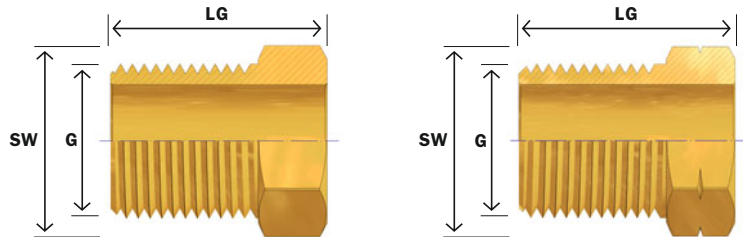
G: Schroefdraad, SW: Sleutelbreedte, LG: Lengte draaibaar draadstuk
